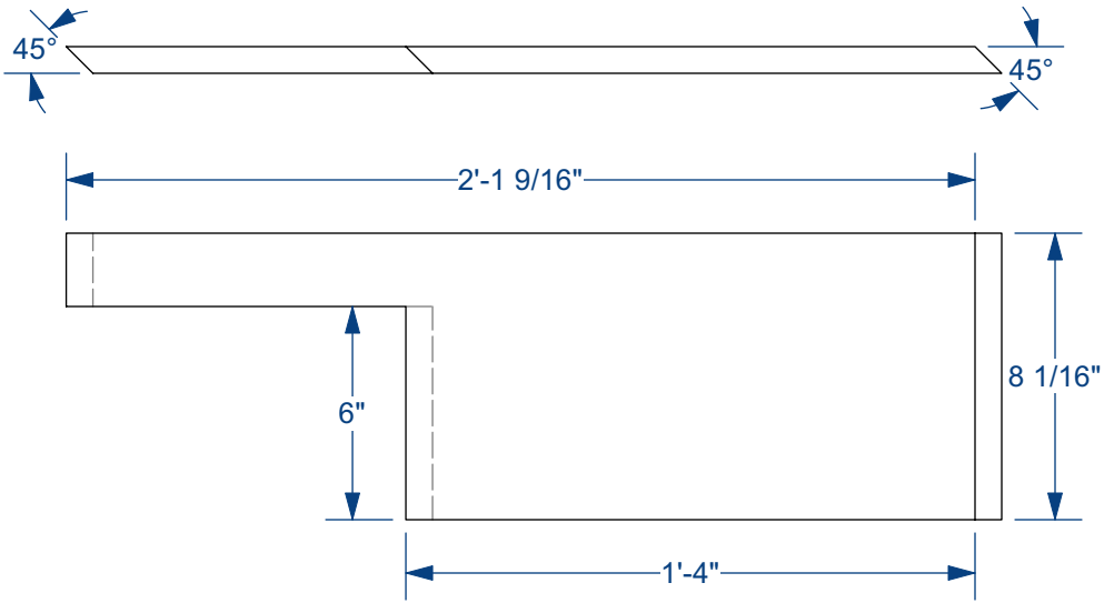
PLYWOOD BOTTOM END PLATE SCALE: 2" = 1'-0"
