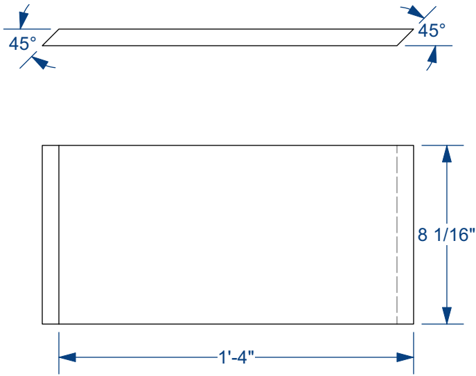
PLYWOOD TOP END PLATE SCALE: 2" = 1'-0"
