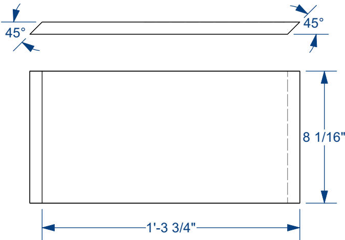
PLYWOOD END PLATE SCALE: 2" = 1'-0"
