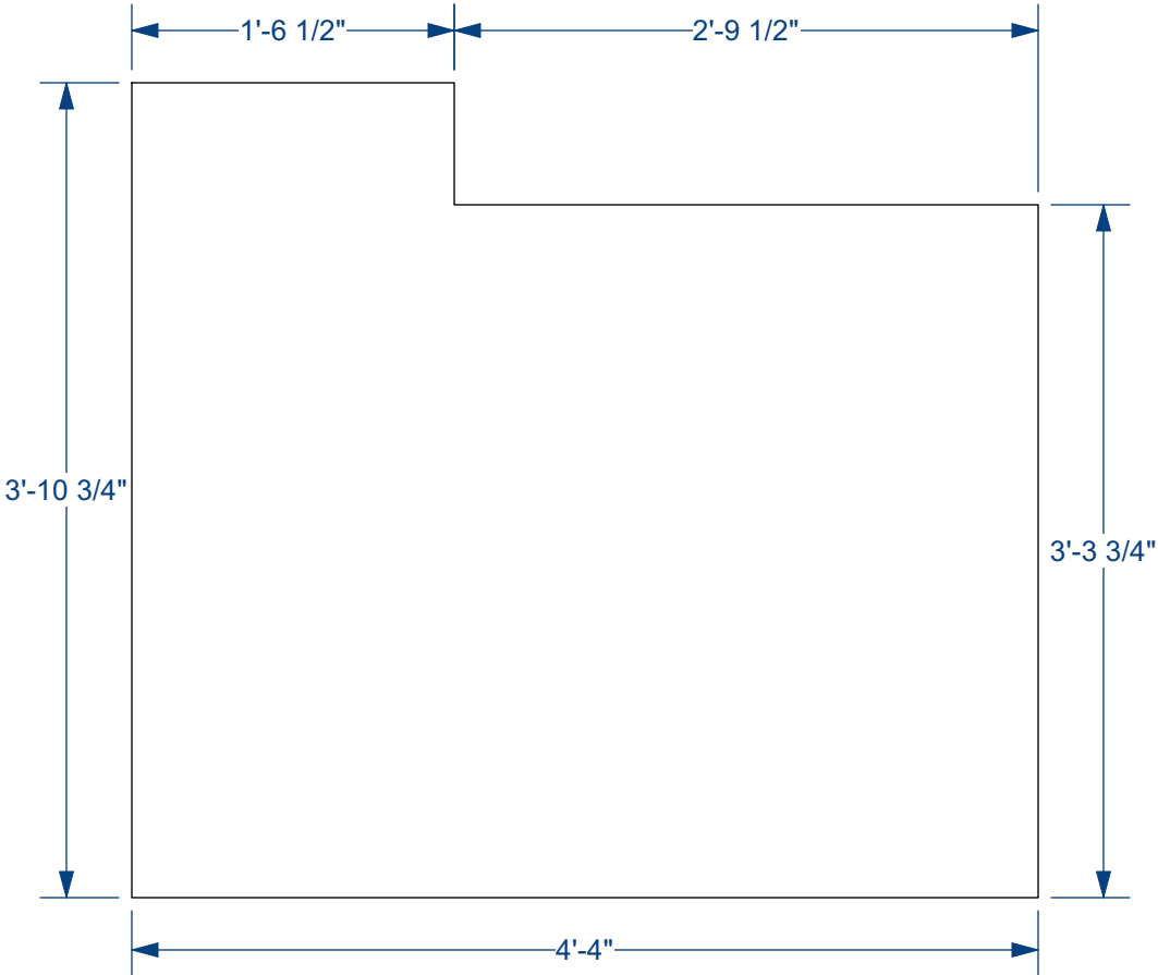
FACE J (R&R)
