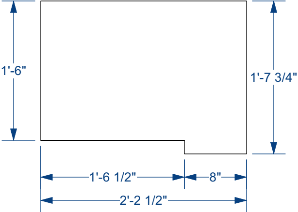
FACE G (R&R)
